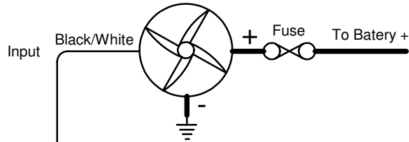
GP1 PWM Fan
